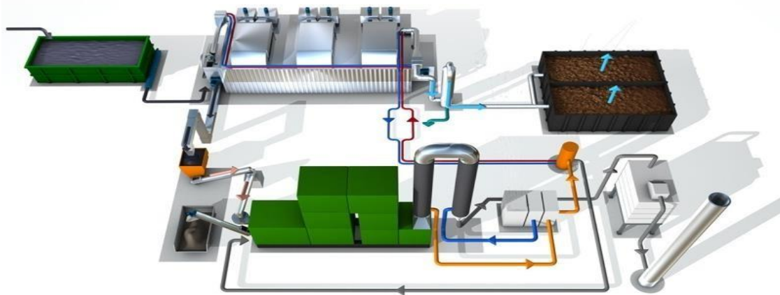
Abbildung 12. HUBER-Schlammwässerungssystem (Quelle: HUBER SE).
