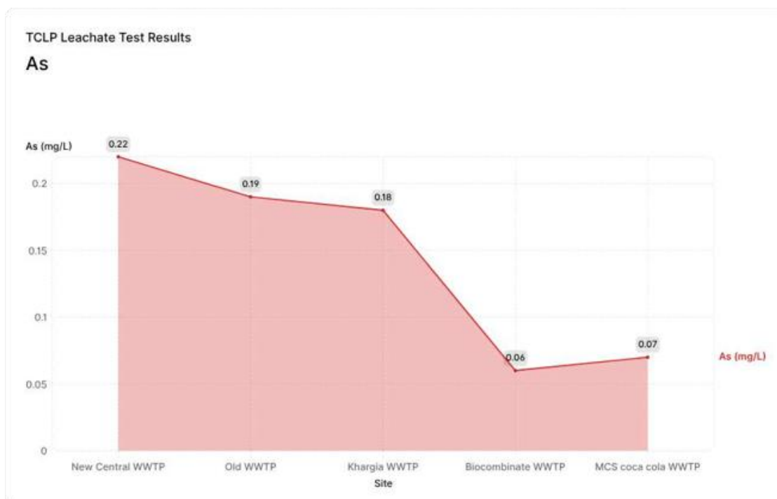
Grafik 1. TCLP Auslaugungstesterebnisse-As
