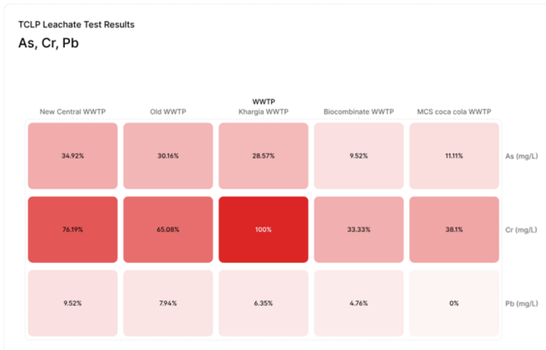
Grafik 5. Ergebnisse des TCLP-Auslaugungstests
