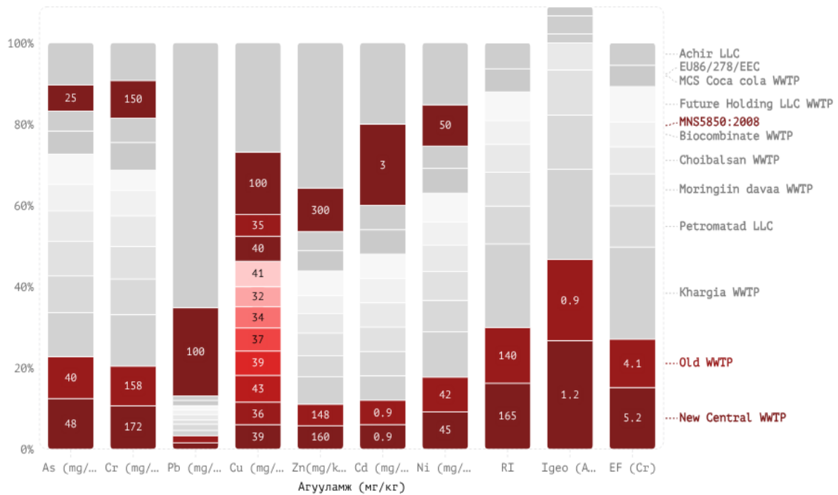
Abbildung 3. Schwermetallanalyse
